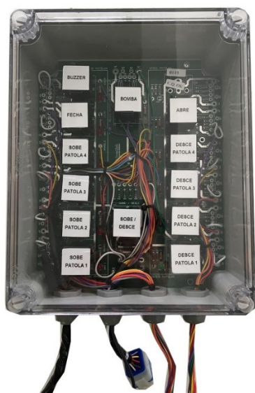
Central de relés
